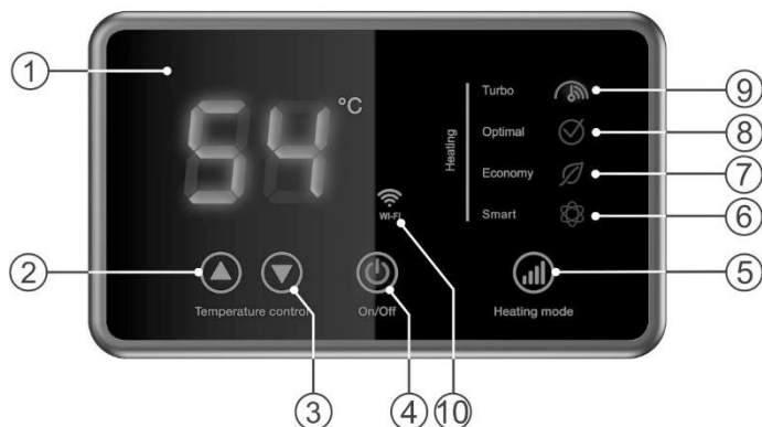
Bild 2. Elektronisches Bedienfeld
